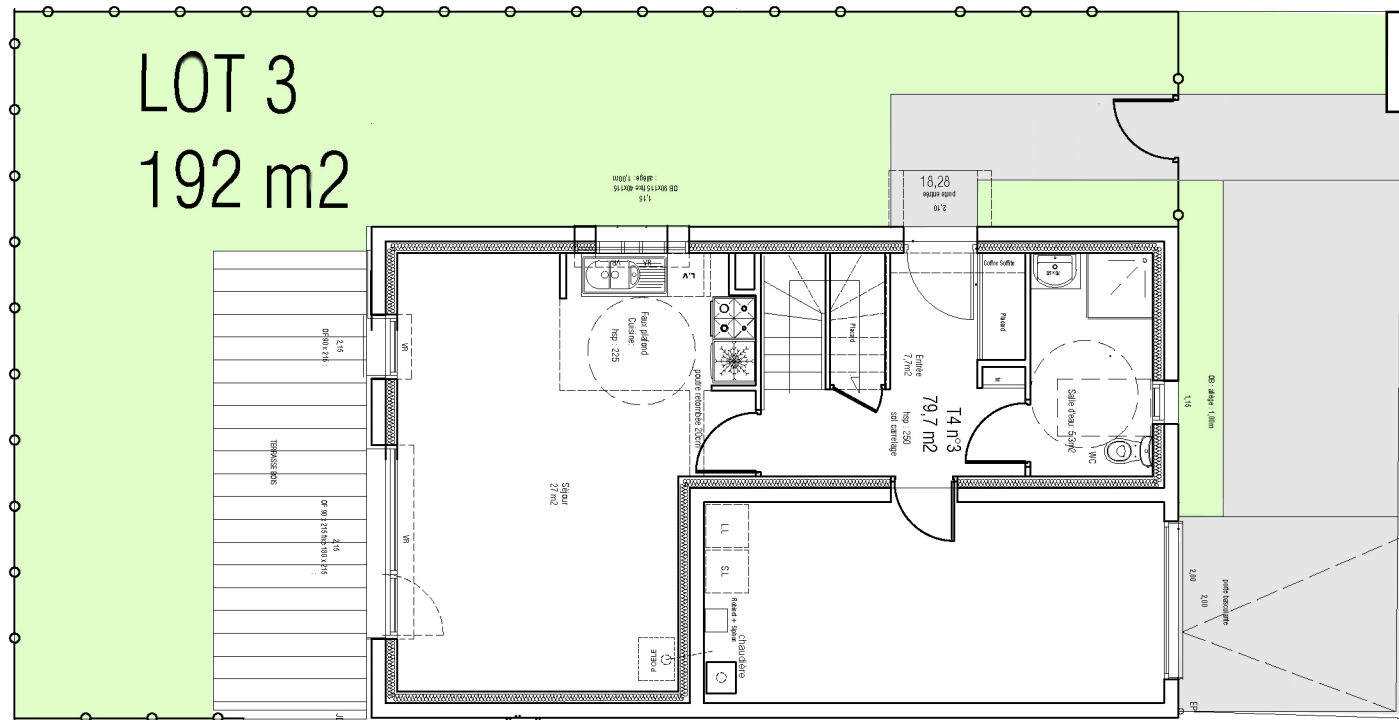
PLAN MASSE RDC DE LA PARCELLE
