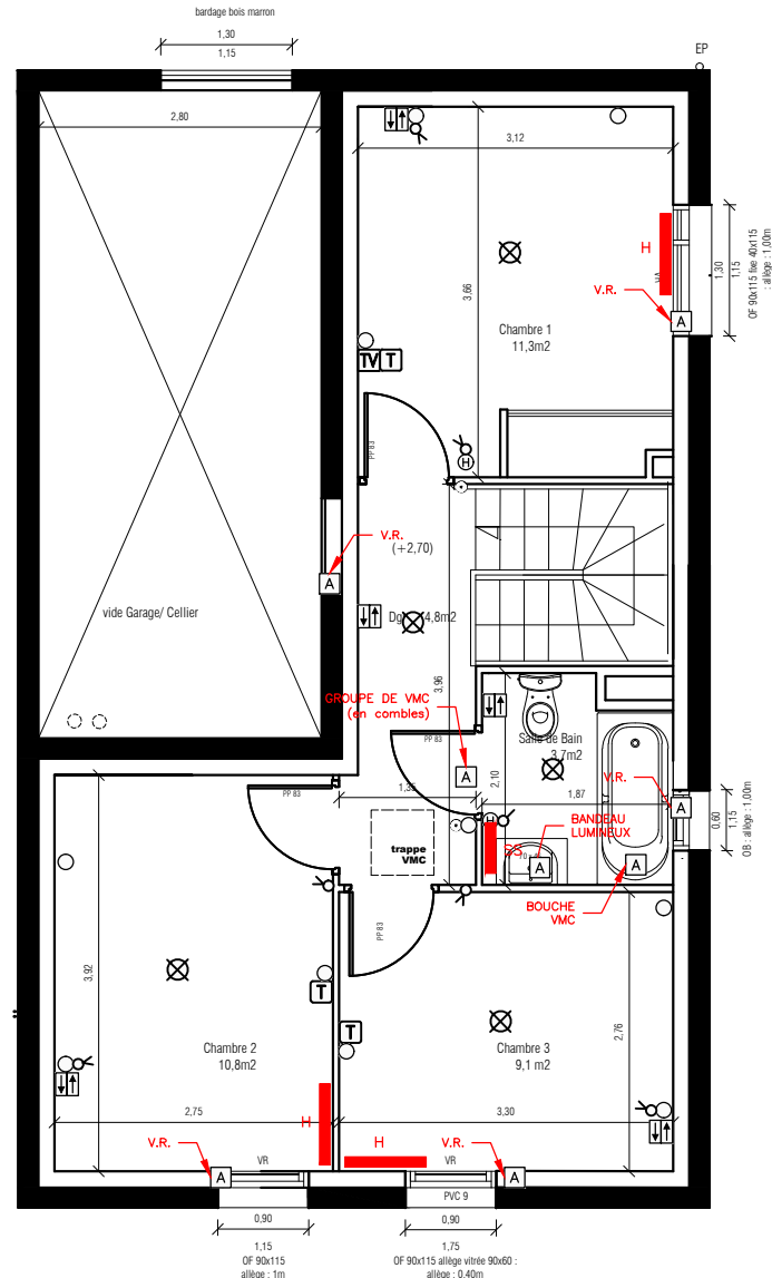
ETAGE 1
